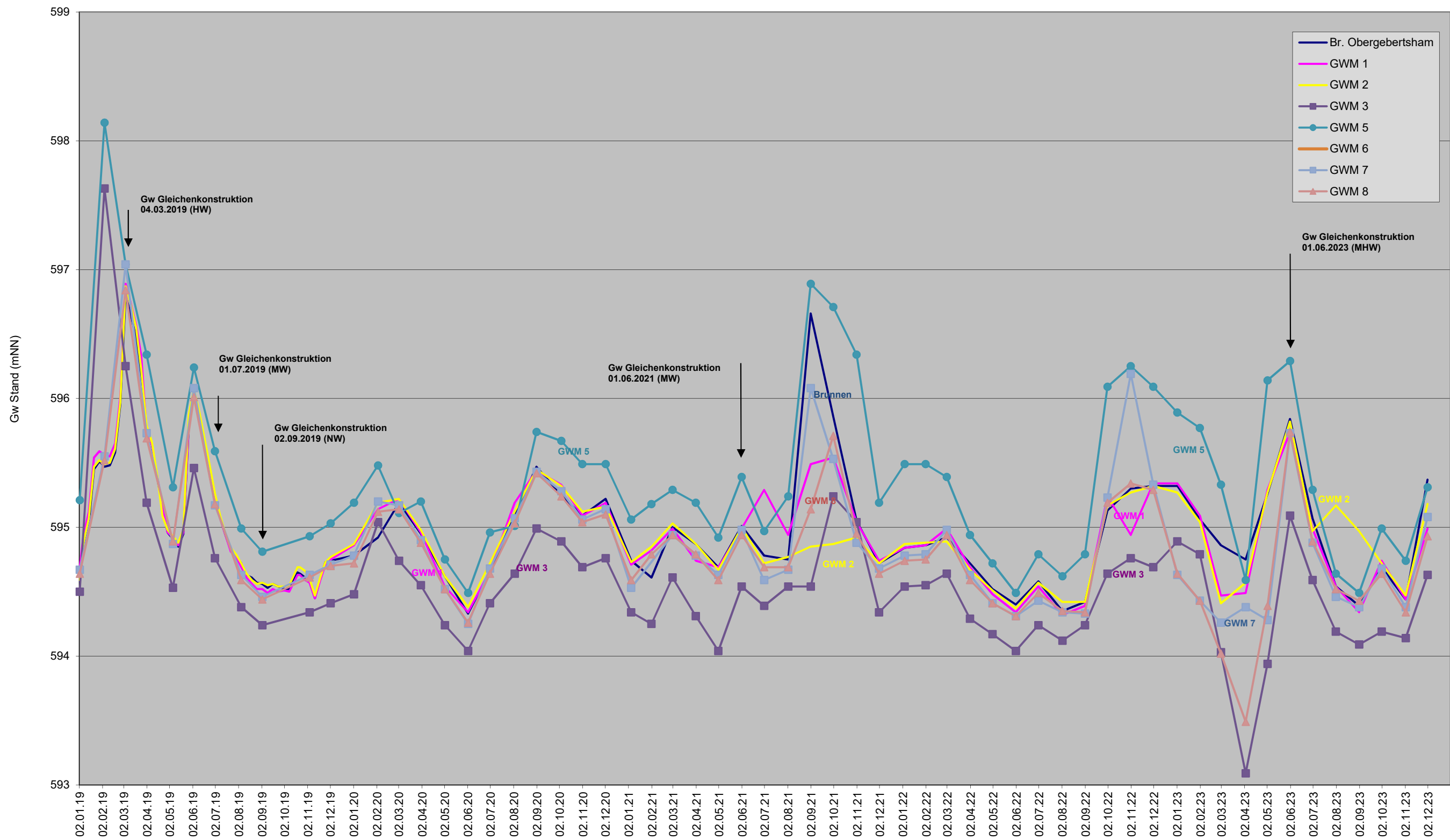
ZV Harpfinger Gruppe Ganglinien des Ruhegrundwasserspiegels im Brunnen Obergebertsham und den Grundwassermeßstellen bei den Stichtagsmessungen des Zweckverbandes Harpfinger Gruppe
